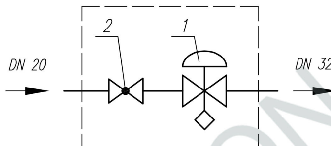
Принципиальная схема
